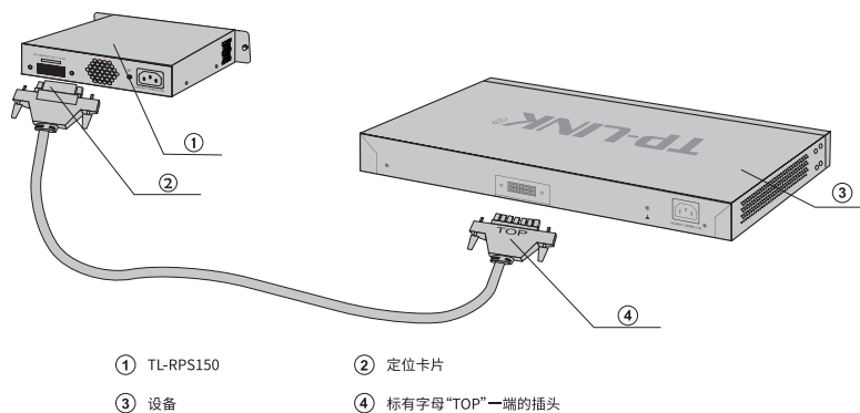
图3-5 连接设备和TL-RPS150示意图
