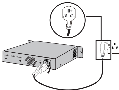
图3-6 TL-RPS150连接电源线示意图
